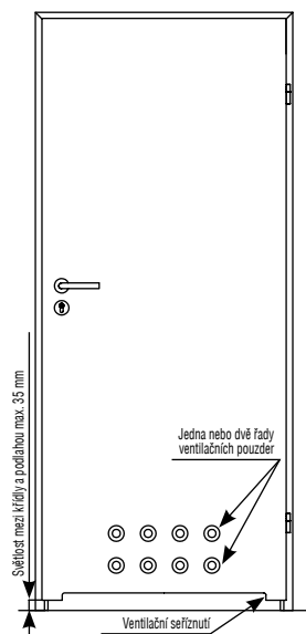
křídlo SEMPRES „80“ s ventilační mezerou
