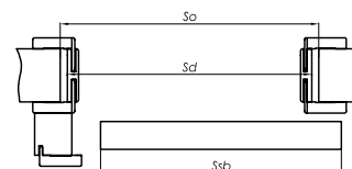
posuvné dveře - nástěnný systém s tunelovou zárubeň ZN
