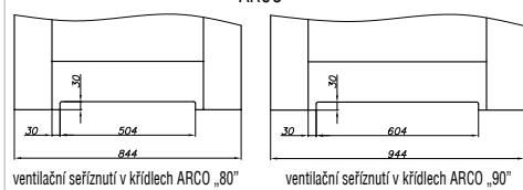
ventilační seřiznutí v křídlech ARCO „80“
