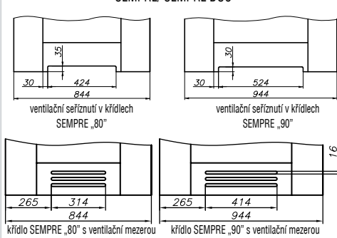
ventilační mezera v křídlech z kolekce SEMPRES - příplatek 589
