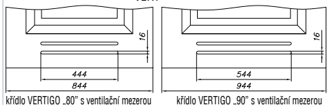
křídlo VERTIGO „80“ s ventilační mezerou
