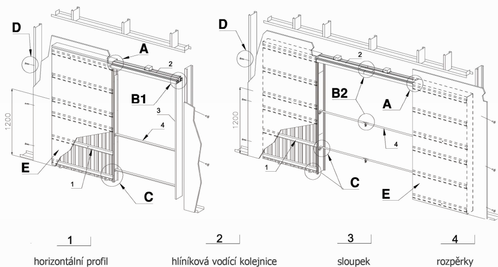
PANORAMA SDK - dvojkřídlé dveře
